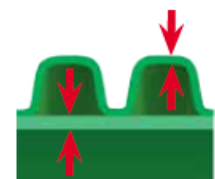
vnitřní stěna - min. 4mm
